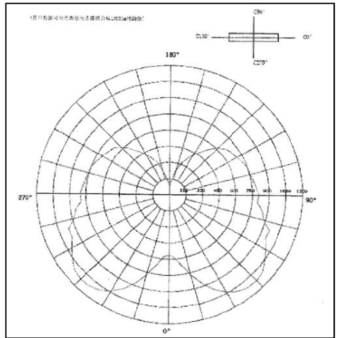
配光曲線(当社の器具による測定値)
